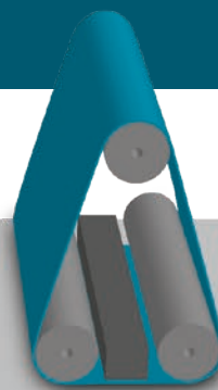
Schleifschuh pneumatisch oder segmentiert
